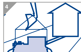
Posadzić zbiornik w wykopie
